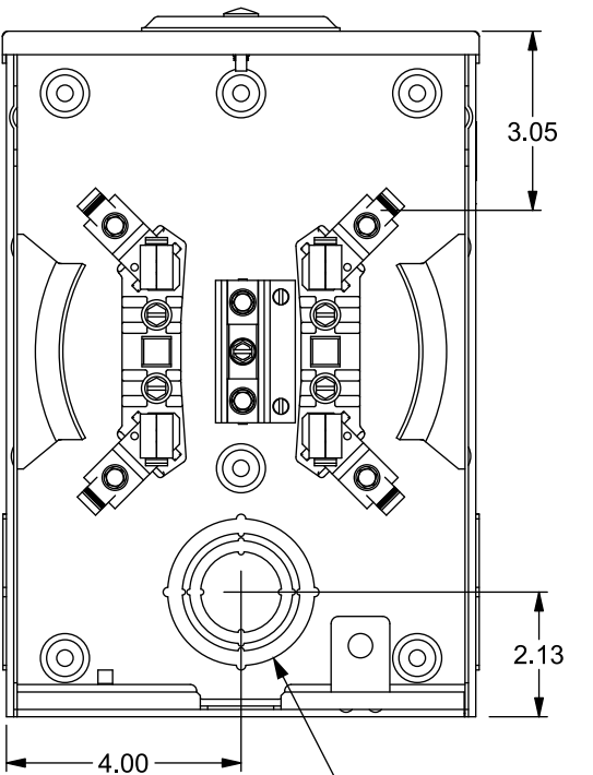
1", 1-1/4", 1-1/2", 2" KO
